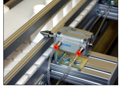
Escapement Gates
